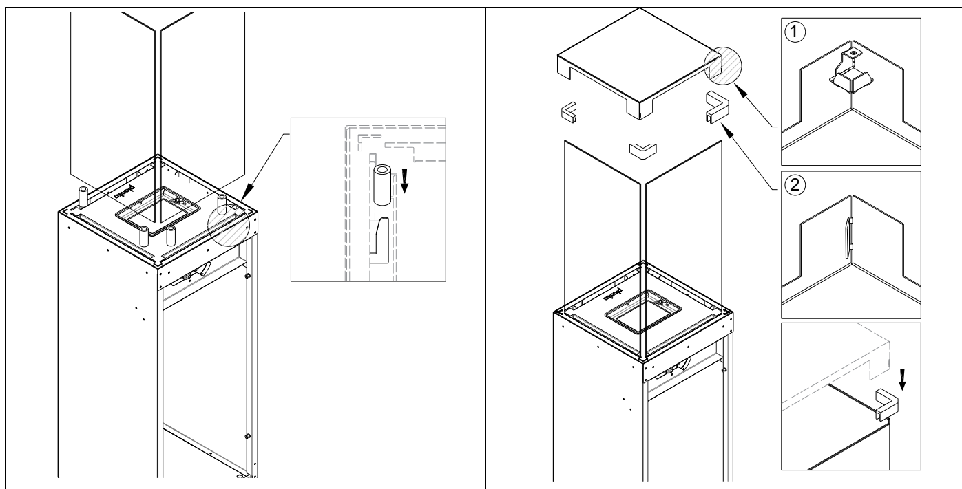
Fig. 5 – Montering av glaset i spåren och metallhuv på glaset
