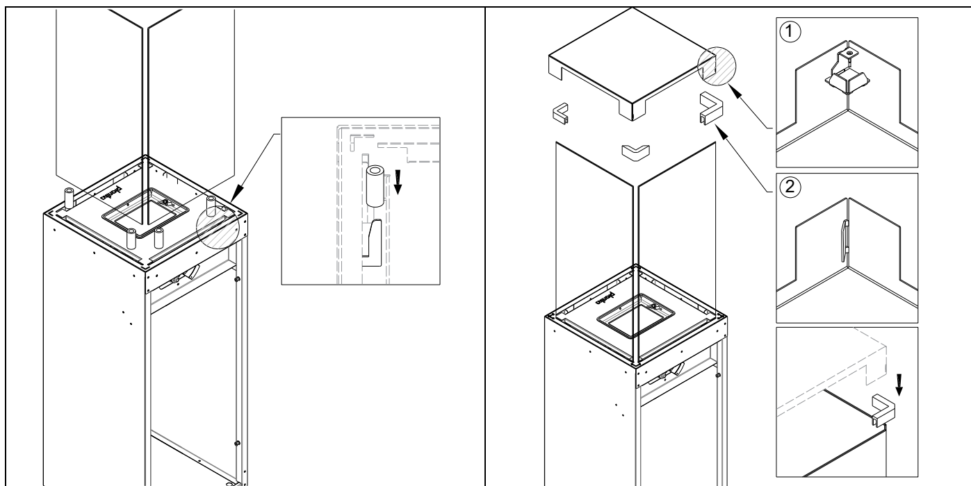
Rys. 5- Montaż szyby w szczelinach i metalowego kaptura na szybie
