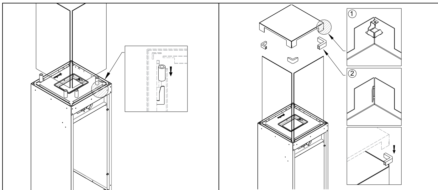
Abb. 5: Einbau des Glases in die Schlitze und der Metallhaube auf dem Glas
