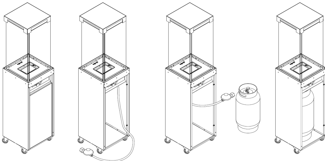
Fig 7- Installation de la bouteille de gaz
