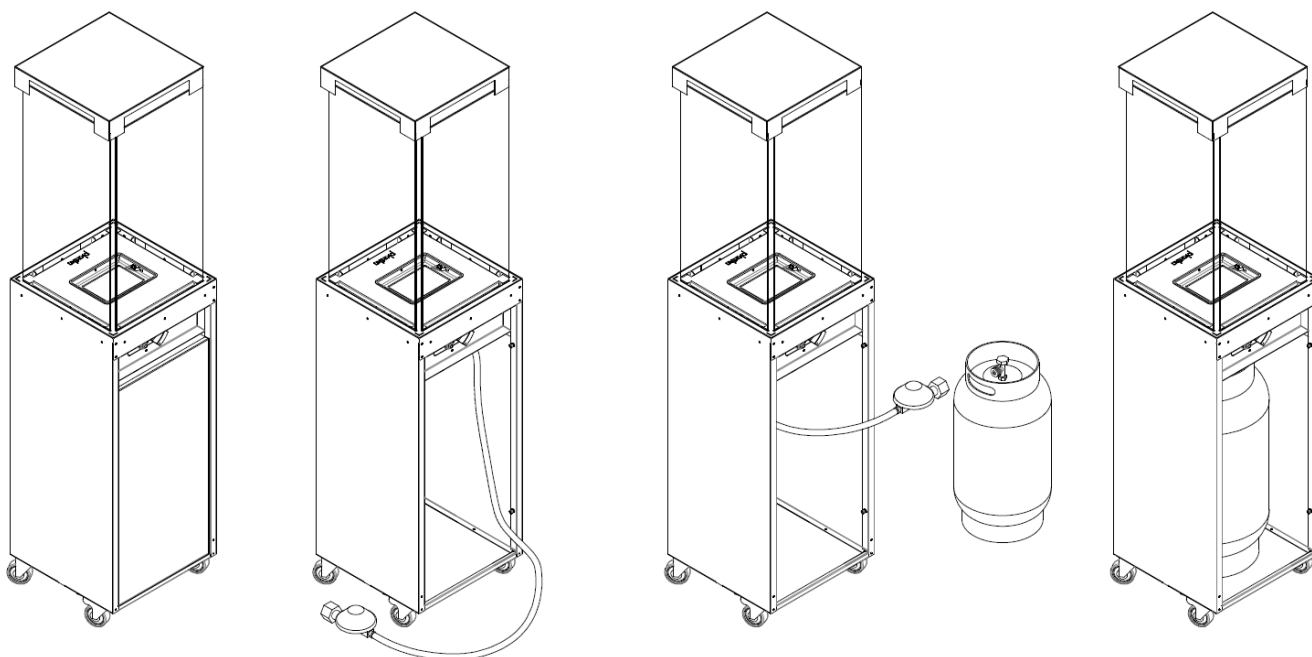
Fig. 6 – Installation av gasflaska
