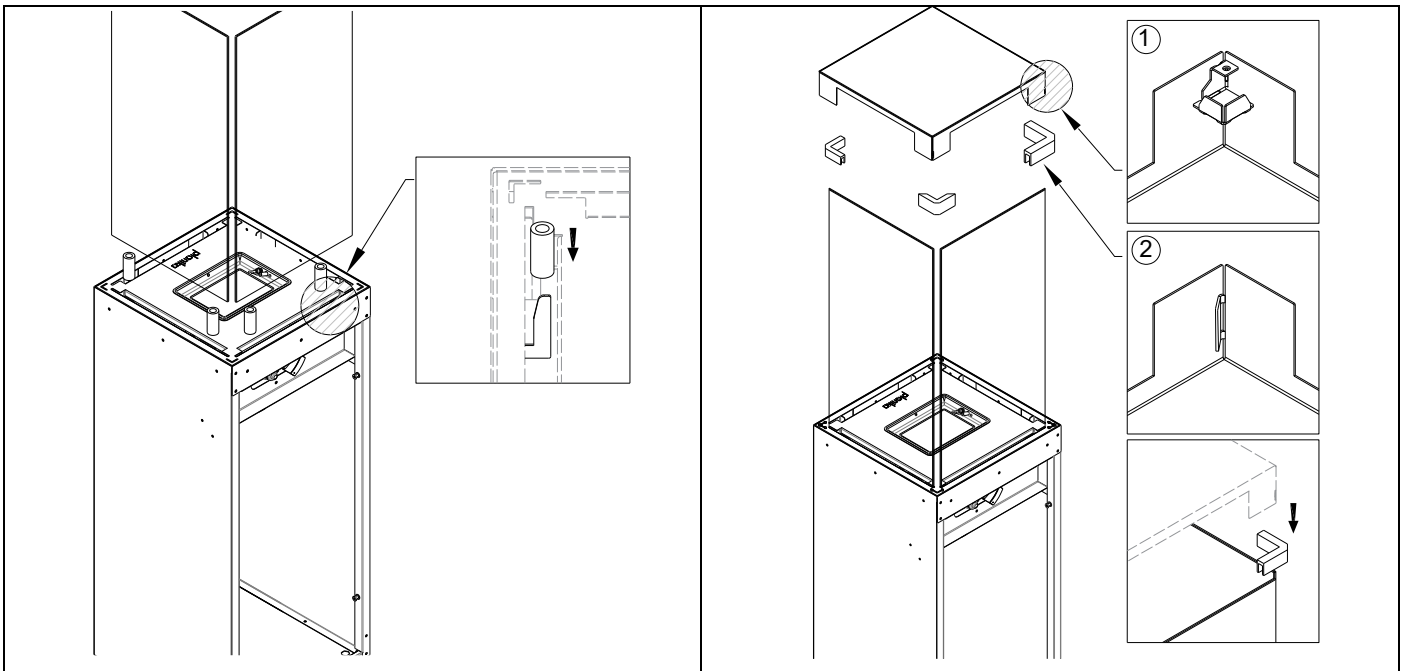
Fig. 5 – Installatie van het glas in de sleuven en de metalen kap op het glas
