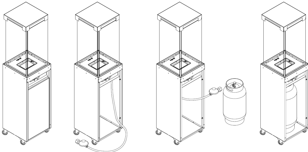
Fig. 6 – Installatie van de gasfles
