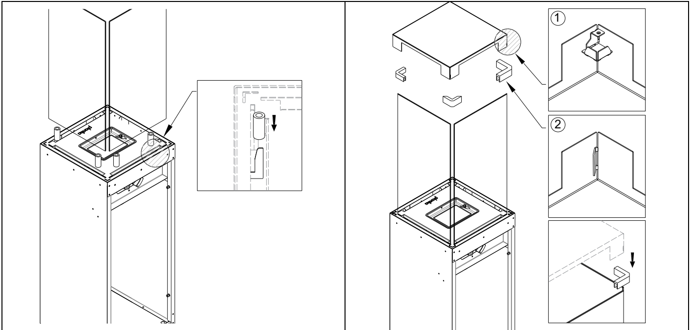
Fig 5- Installation de la vitre dans les fentes et du capot métallique sur la vitre
