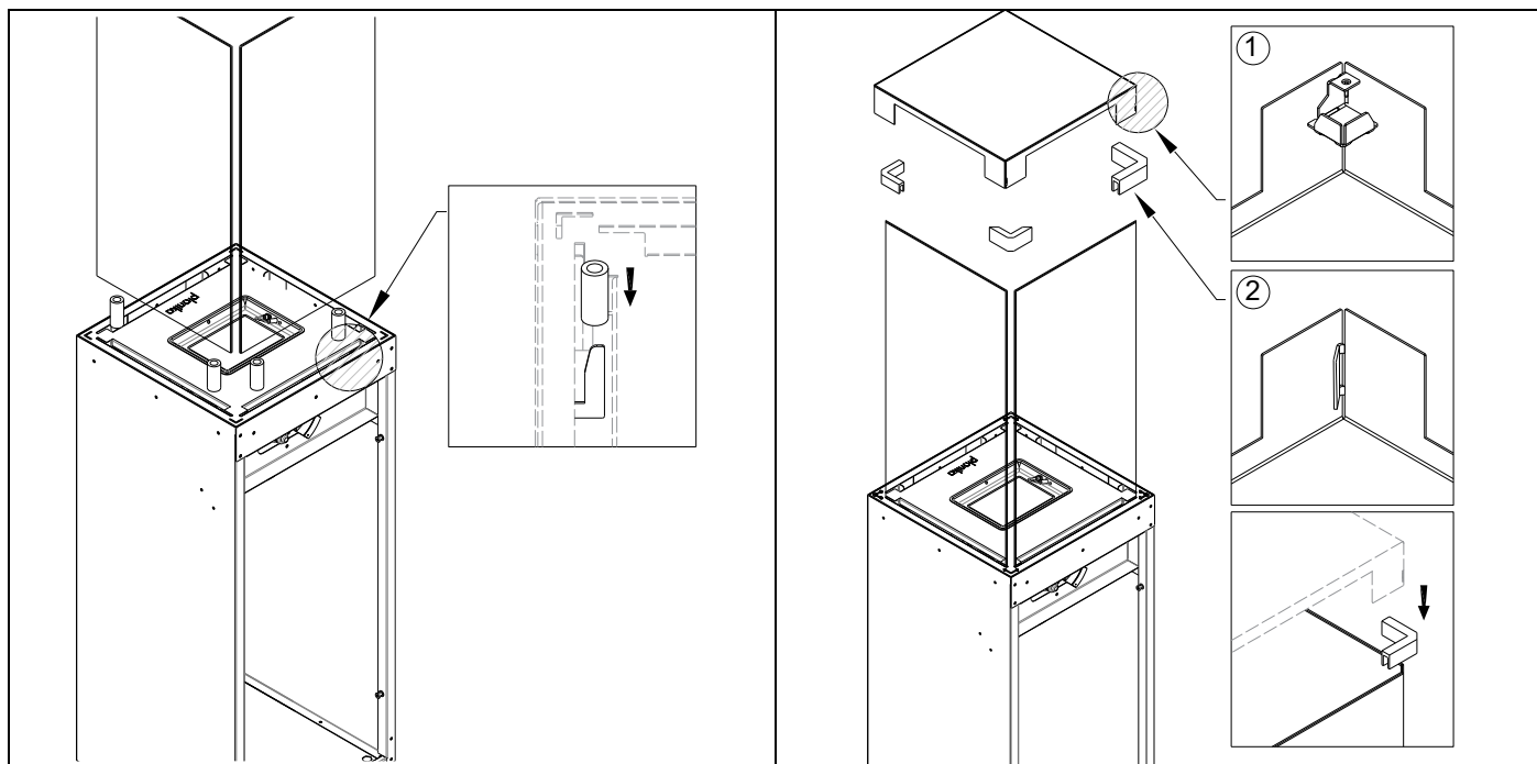
Fig 5- Installazione del vetro nelle fessure e della calotta metallica sul vetro
