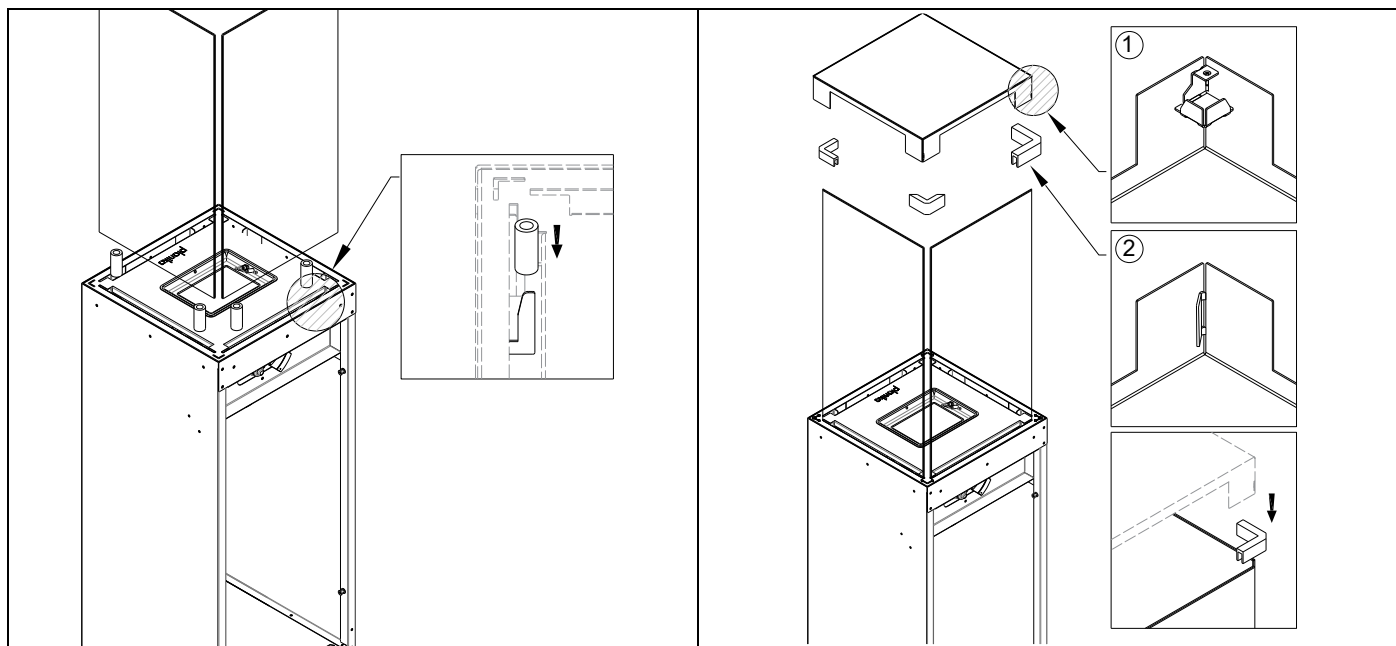
Fig 5- Instalación del cristal en las ranuras y de la campana metálica sobre el cristal
