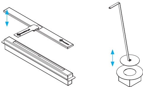
Rys. 3. Biopojemniki z dedykowaną przesłoną służącą do wygaszania palnika: a) Flat, b) Tango Fig. 3. Bio-fuel canisters with the dedicated burner snuffer: (a) Flat; (b) Tango
